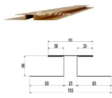
З'єднувальна планка (Фасадна, Сайдинг)
