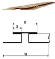
З'єднувальна планка (Фасадна, Сайдинг)
